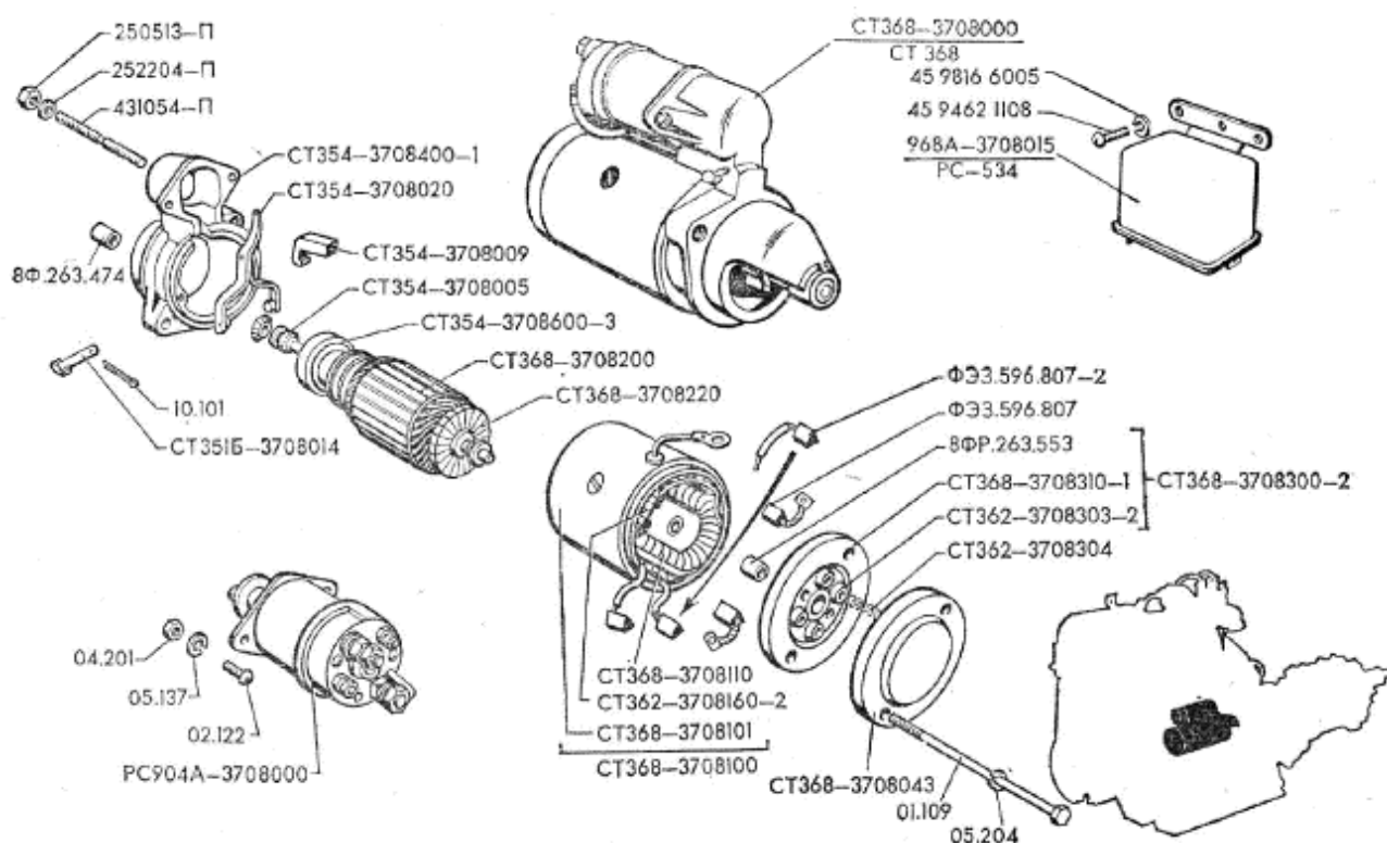
Рис.58. Стартер и включатель стартера 1 von 2
