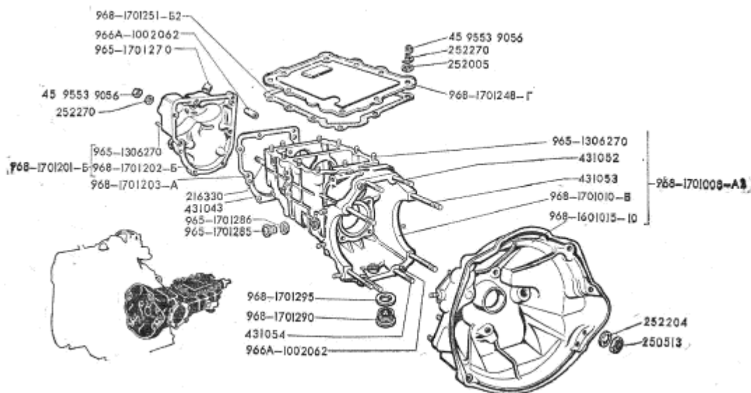
Рис.32. Картеры коробки передач и сцепления
