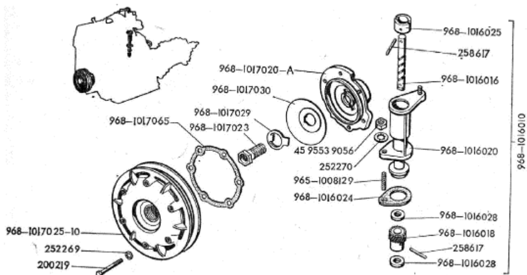
Рис.16.Привод распределителя зажигания и маслоочиститель
