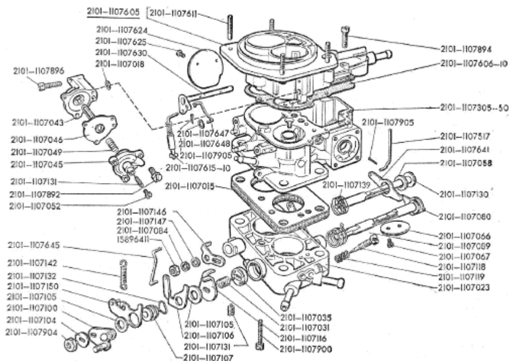
Рис.22. Детали карбюратора ДААЗ 2101-20 1 von 3
