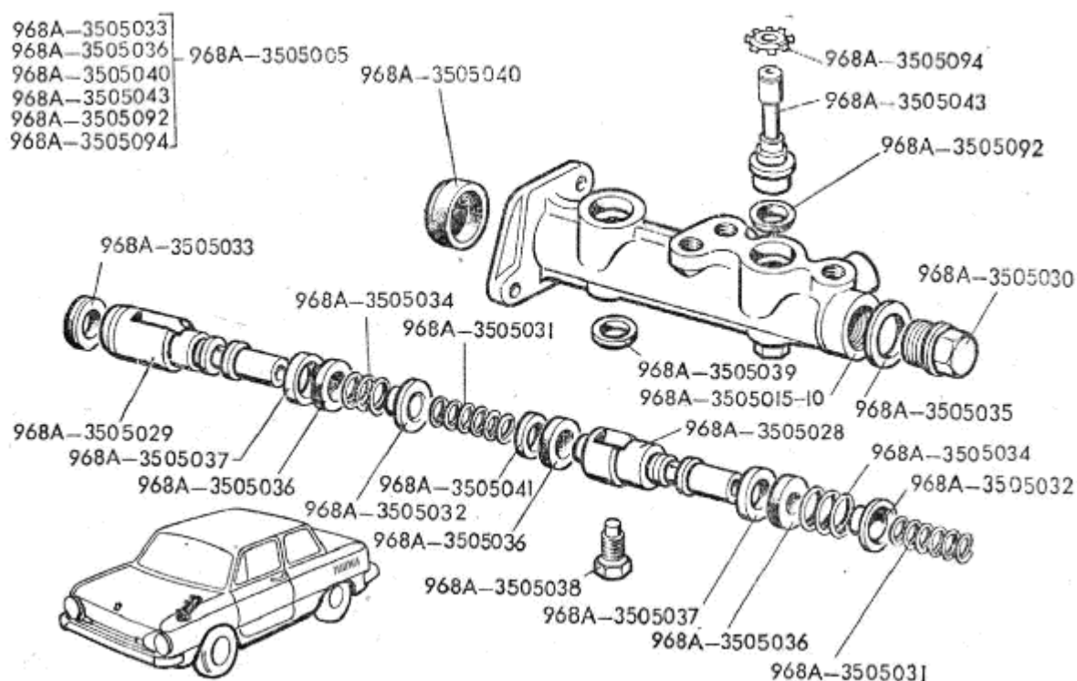
Рис.53. Детали главного тормозного цилиндра
