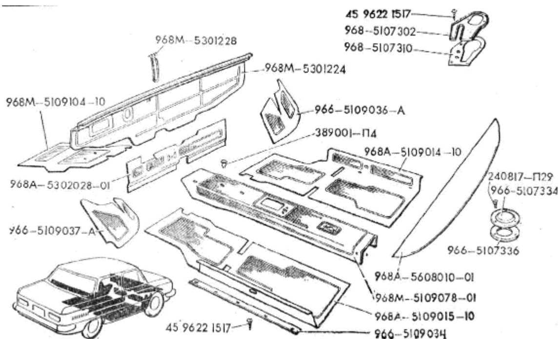
Рис.65. Коврики пола и крышки люков
