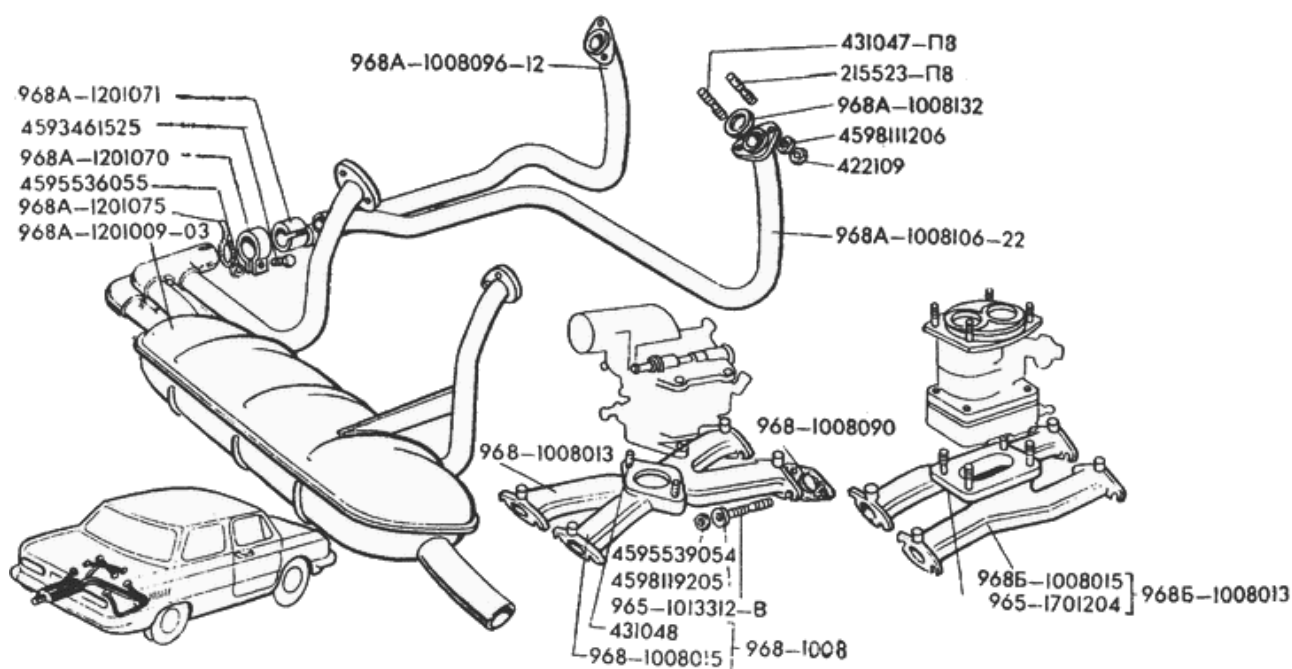
Рис.13. Впускной и выпускной трубопроводы и глушитель
