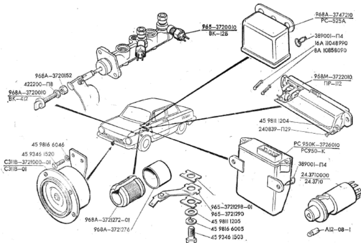
Рис.60. Звуковой сигнал, блок предохранителей, сигнализация аварийная 1 von 2
