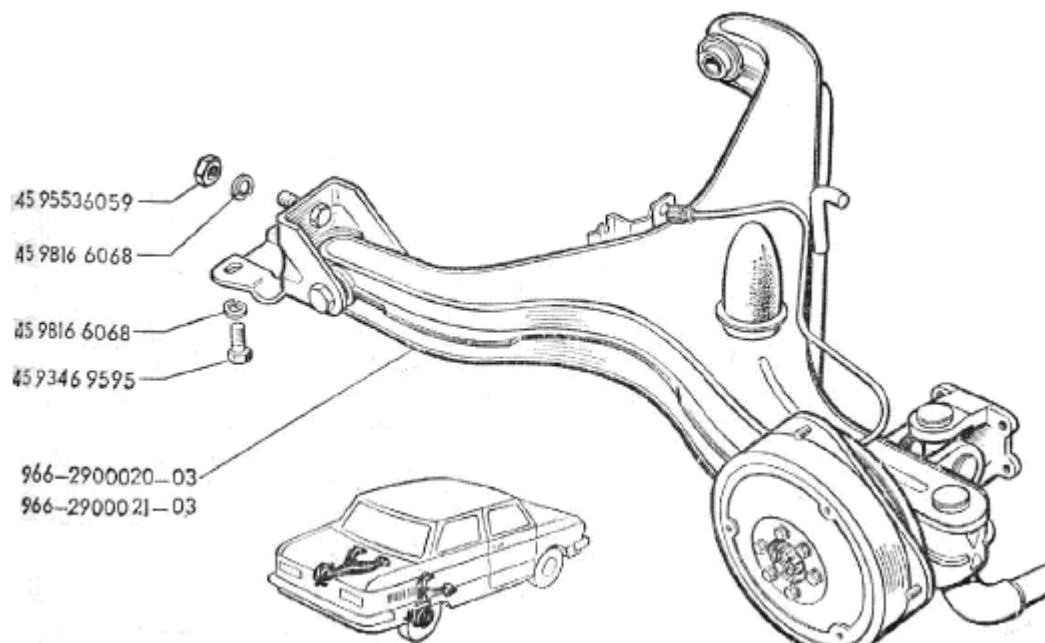
Рис.39. Рычаг задней подвески
