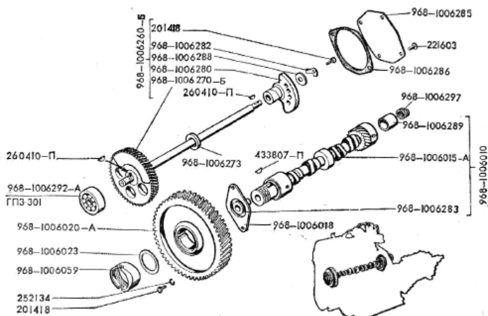
Рис.11. Распределительный и балансирный валы
