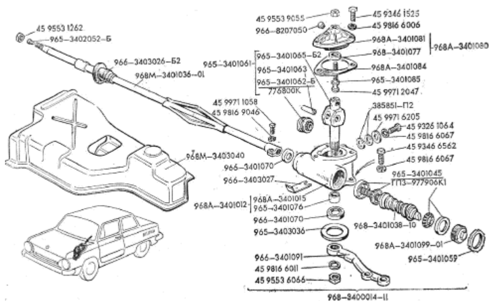
Рис.49. Рулевой механизм 1 von 2
