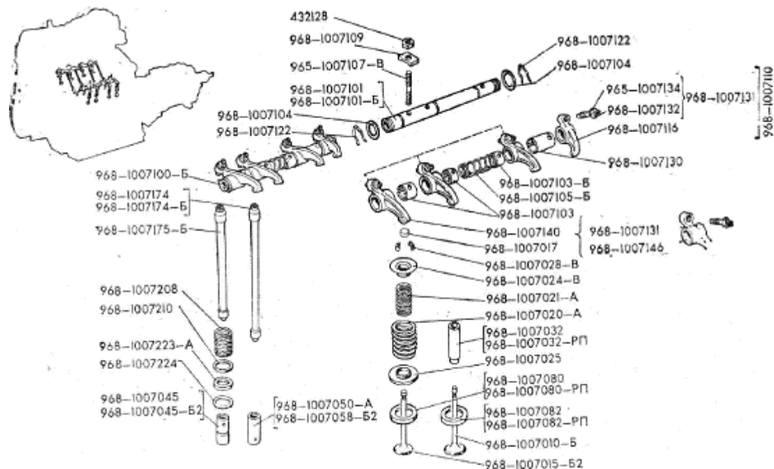
Рис.12. Клапаны и толкатели 1 von 2
