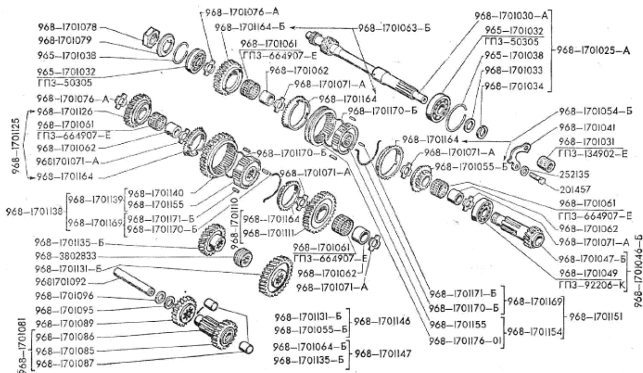
Рис.33. Детали коробки передач 4 von 4
