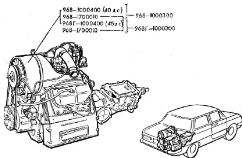
Рис. 5. Силовой агрегат в сборе
