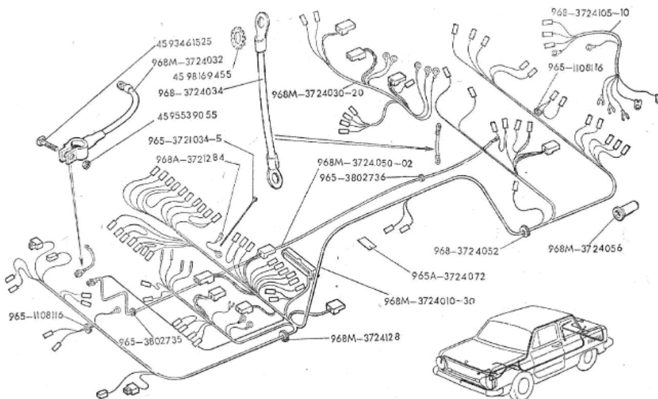
Рис.61. Электропровода
