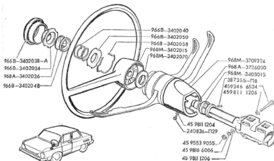
Рис.48. Рулевое колесо и опора вала рулевого механизма
