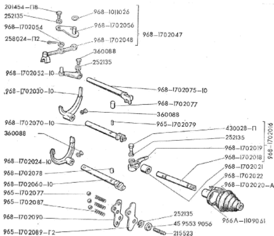
Рис.34. Детали коробки передач 1 von 2
