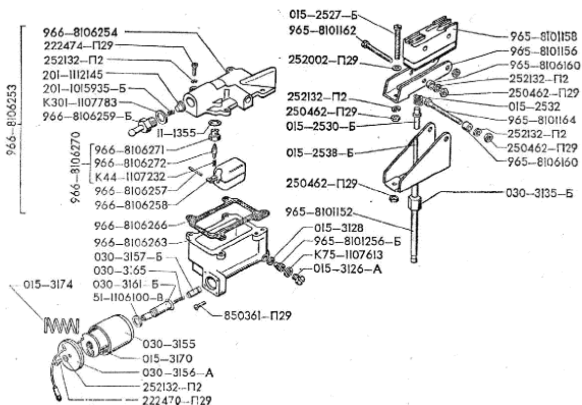
Рис.77. Детали отопительной установки 1 von 2
