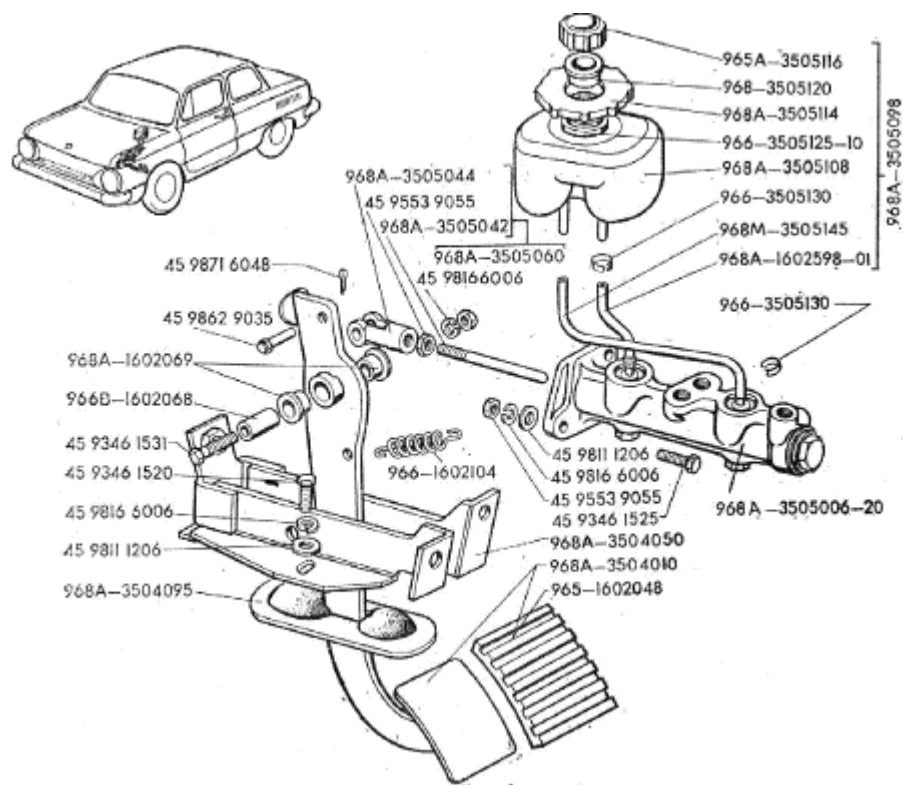
Рис.52. Привод гидравлического тормоза 2 von 2
