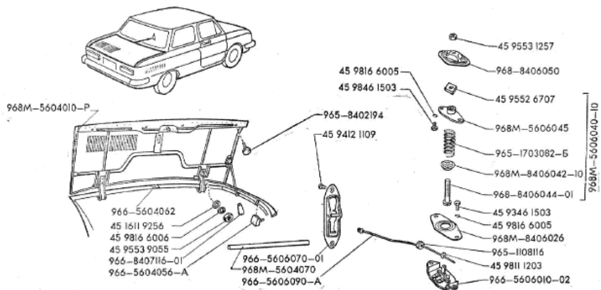
Рис.71. Капот задка
