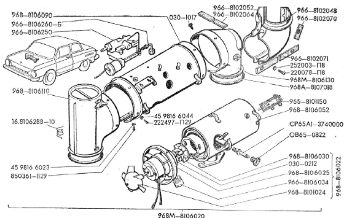
Рис.76. Отопительная установка
