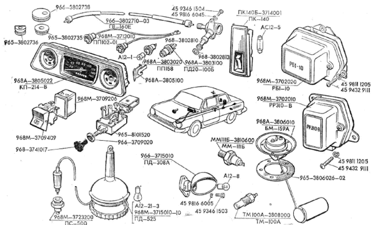
Рис.62. Щиток приборов, датчики и реле 1 von 2
