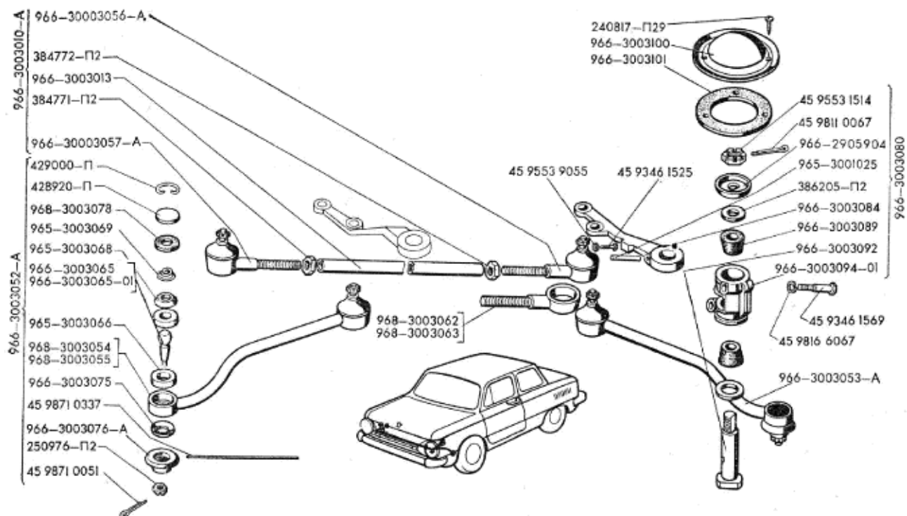
Рис.45. Рулевые тяги и маятниковый рычаг 1 von 2
