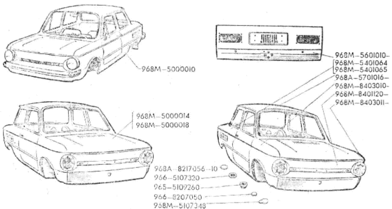
Рис.64. Кузов и его детали
