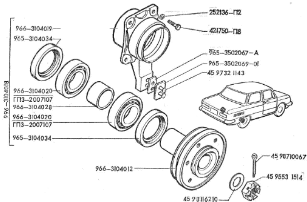
Рис.47. Ступица заднего колеса
