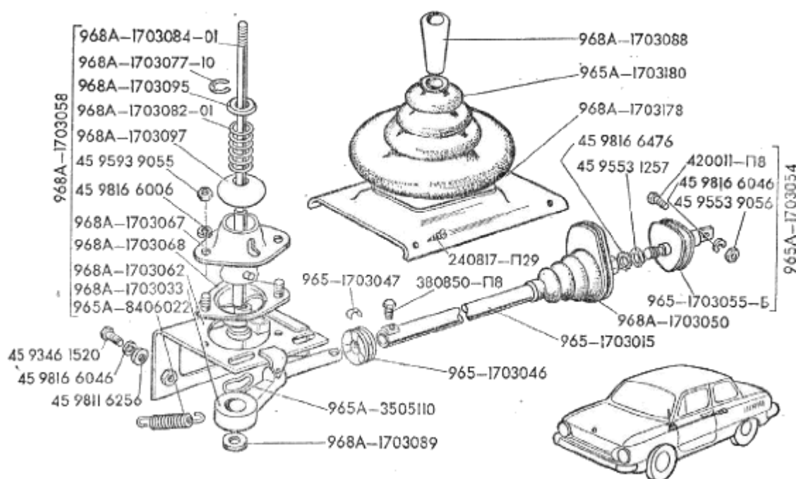
Рис.35. Механизм управления коробкой передач 2 von 2
