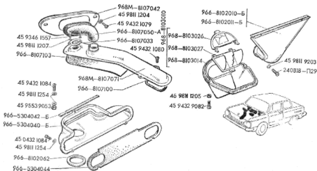
Рис.69. Детали вентиляции кузова
