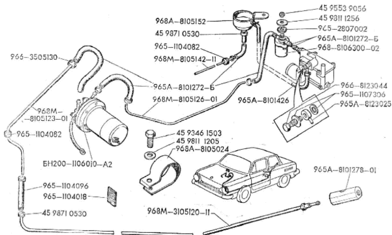
Рис.78. Питание отопительной установки
