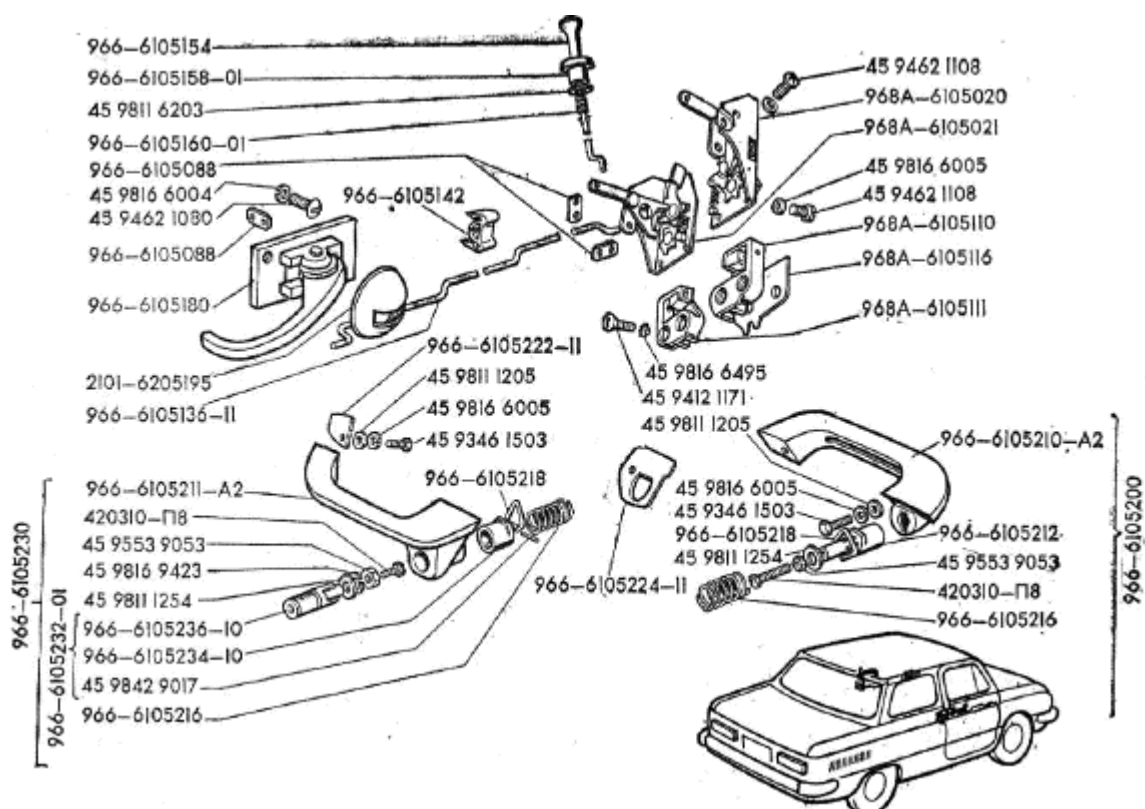
Рис.74. Замок и ручки двери 1 von 2
