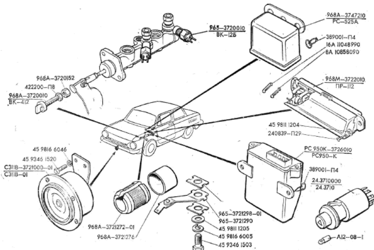
Рис.60. Звуковой сигнал, блок предохранителей, сигнализация аварийная 2 von 2
