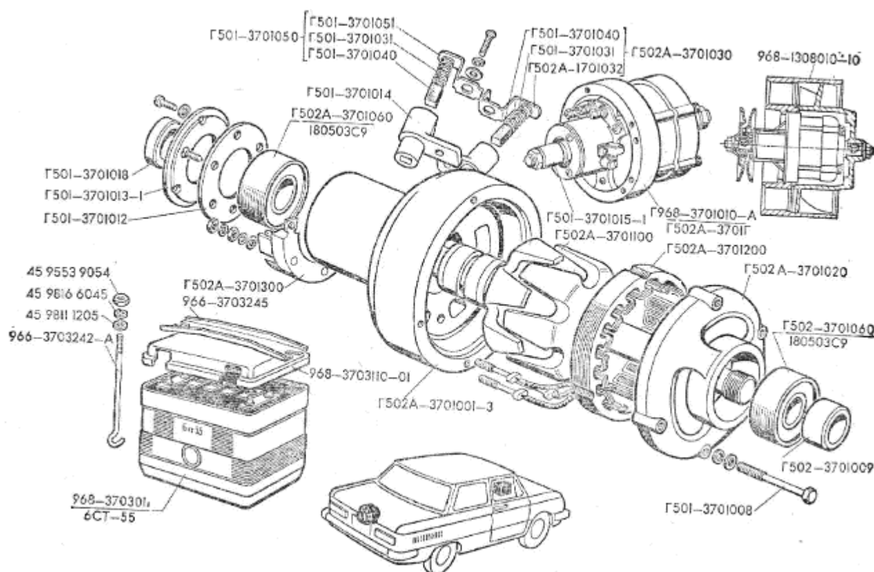
Рис.56. Генератор и аккумуляторная батарея 2 von 2
