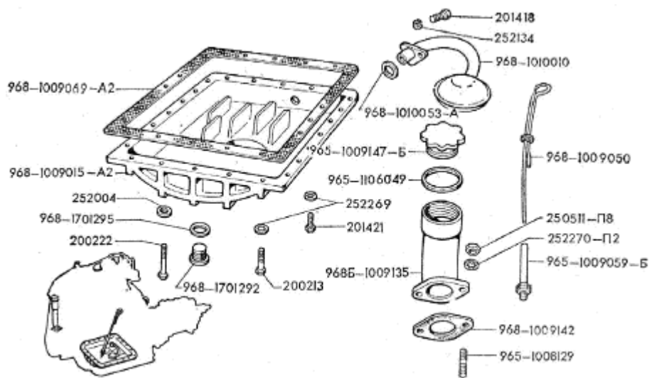
Рис. 14. Картер двигателя и маслоприемник
