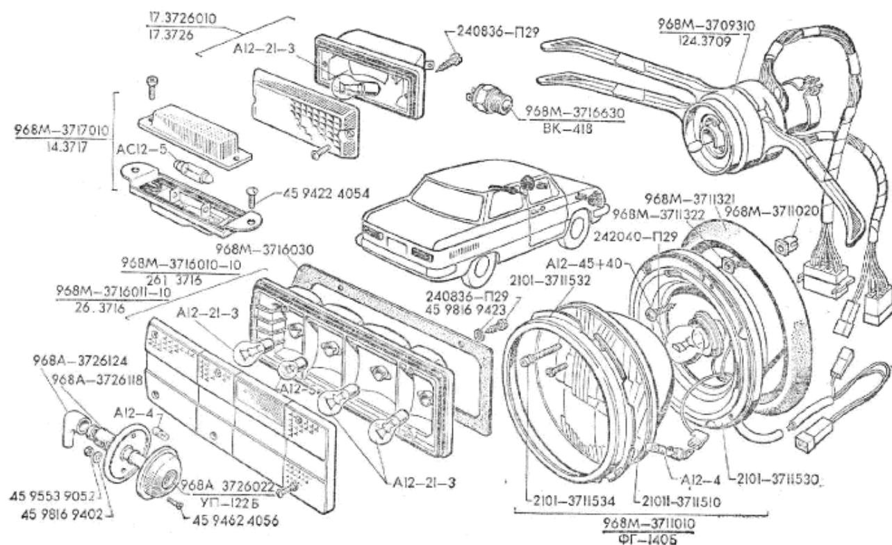
Рис.59. Освещение и световая сигнализации 1 von 2
