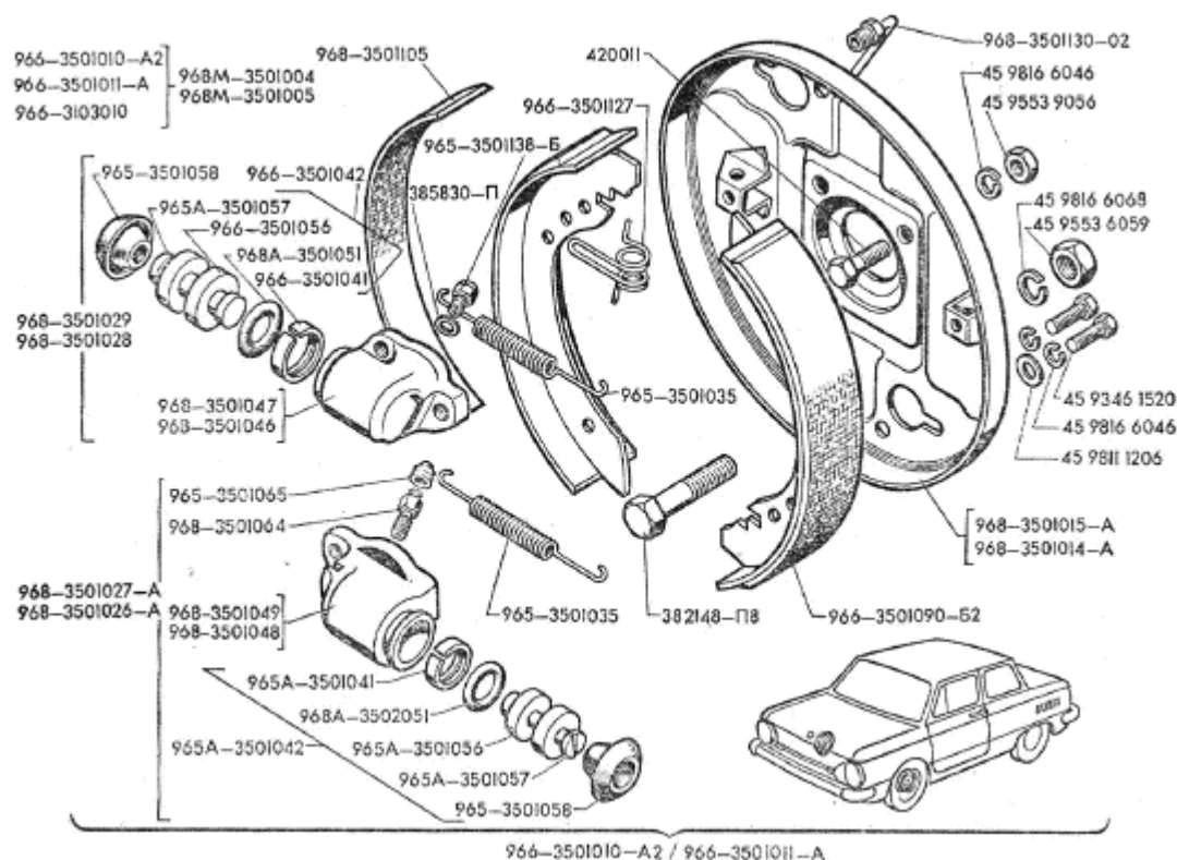
Рис.50. Передний тормоз 2 von 2
