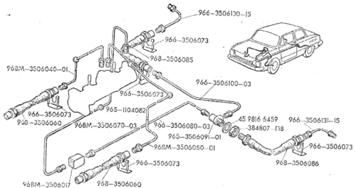
Рис.54. Трубопроводы гидравлического тормоза
