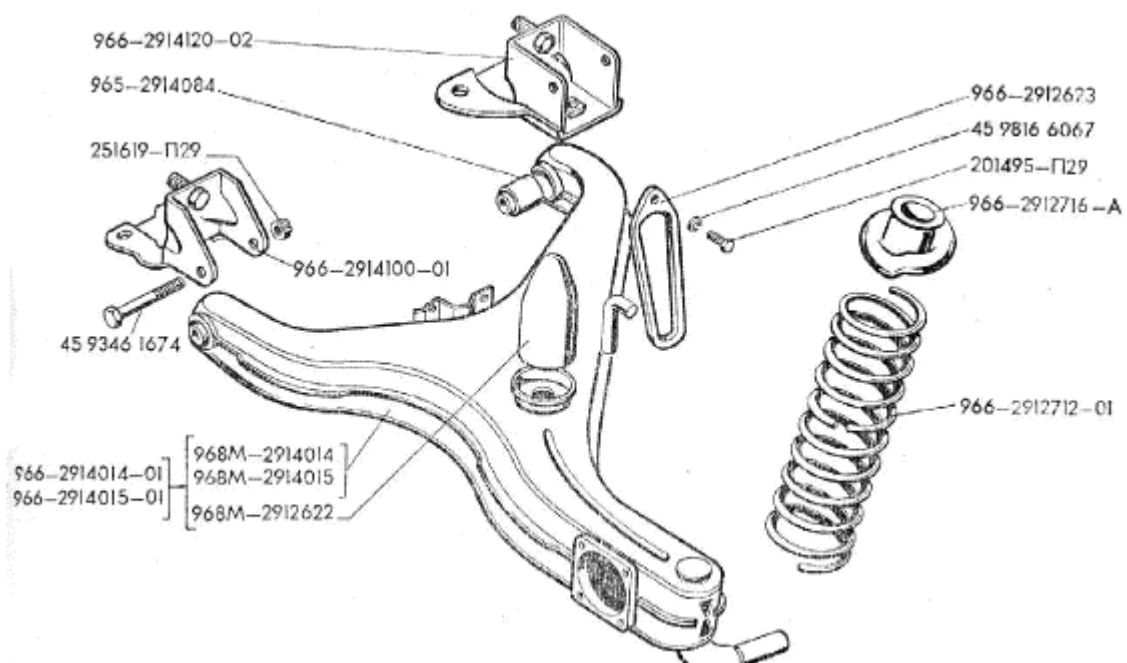
Рис.43. Детали задней подвески
