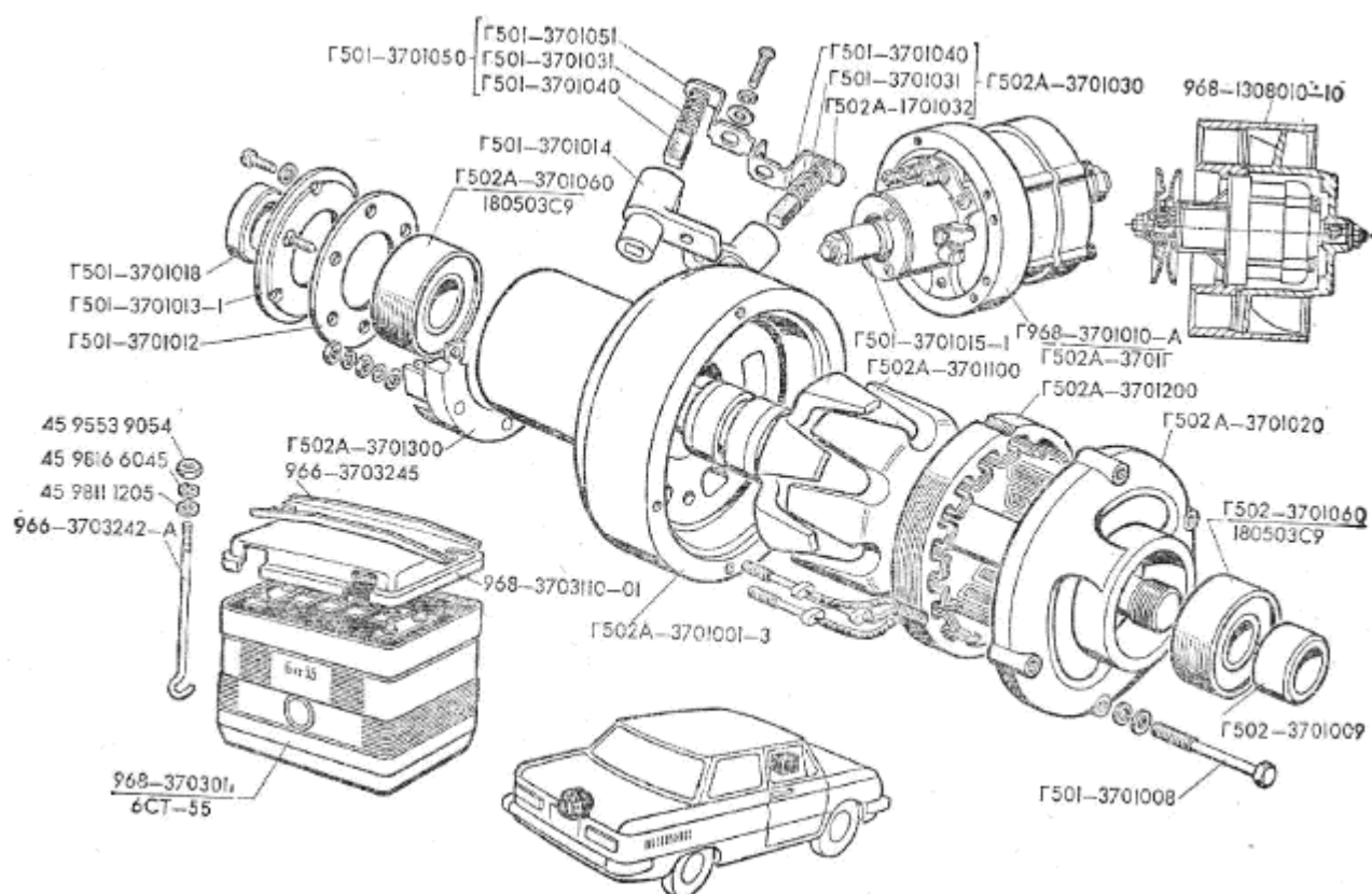
Рис.56. Генератор и аккумуляторная батарея 1 von 2
