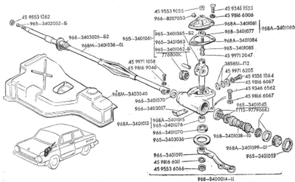
Рис.49. Рулевой механизм 2 von 2
