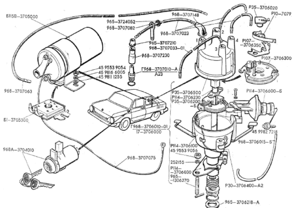
Рис.57. Детали системы зажигания 1 von 2
