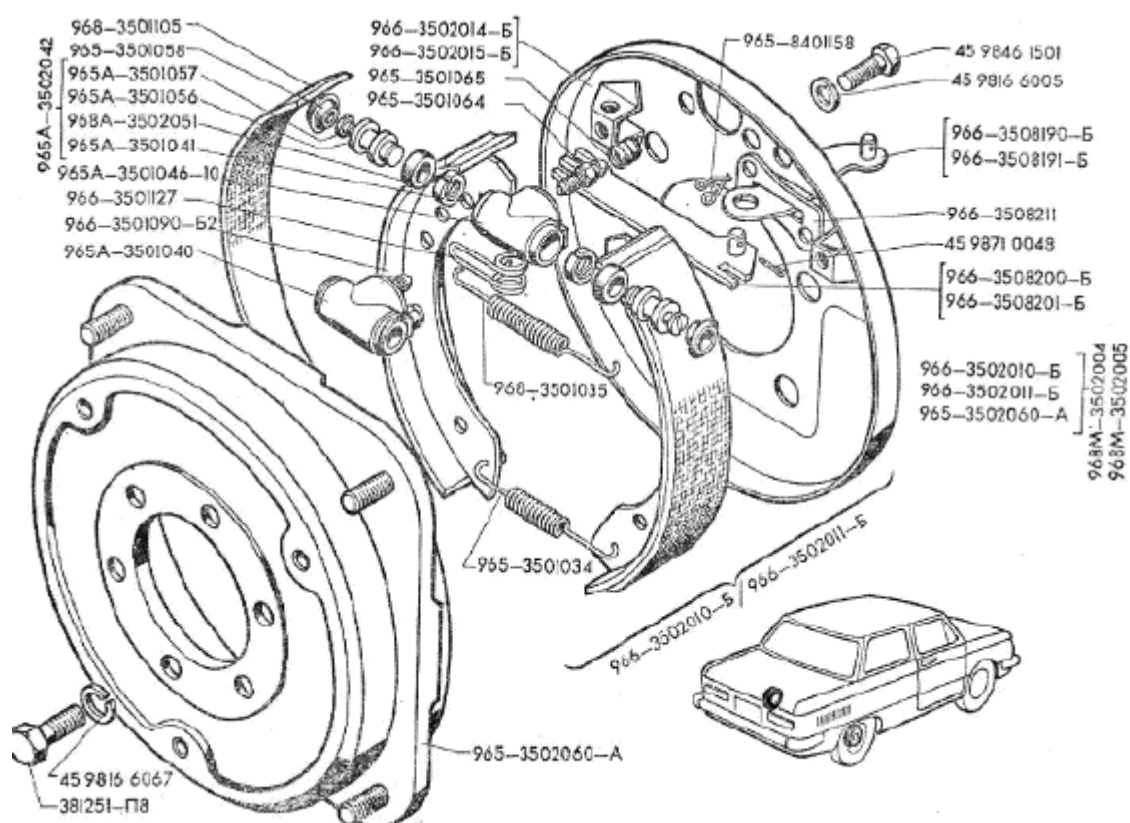
Рис.51. Задний тормоз 2 von 2
