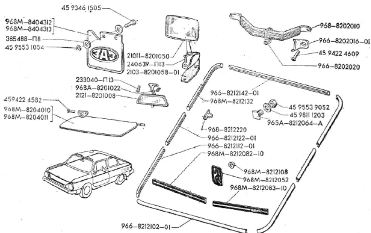
Рис.79. Орнаменты, декоративные надписи и принадлежности кузова
