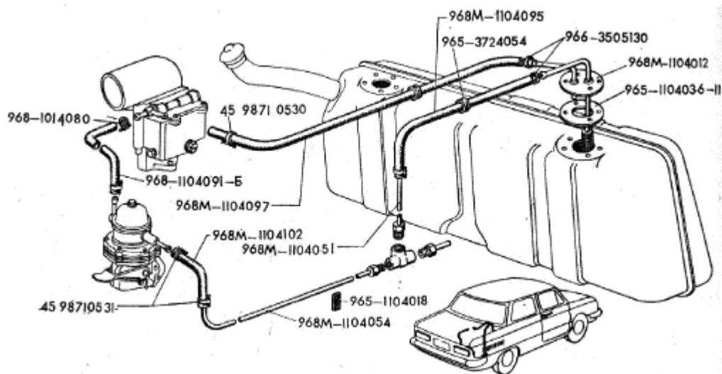
Рис.18. Топливные трубопроводы
