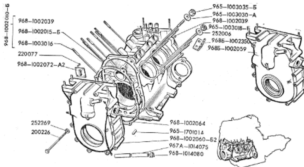
Рис. 7. Картер коленчатого вала
