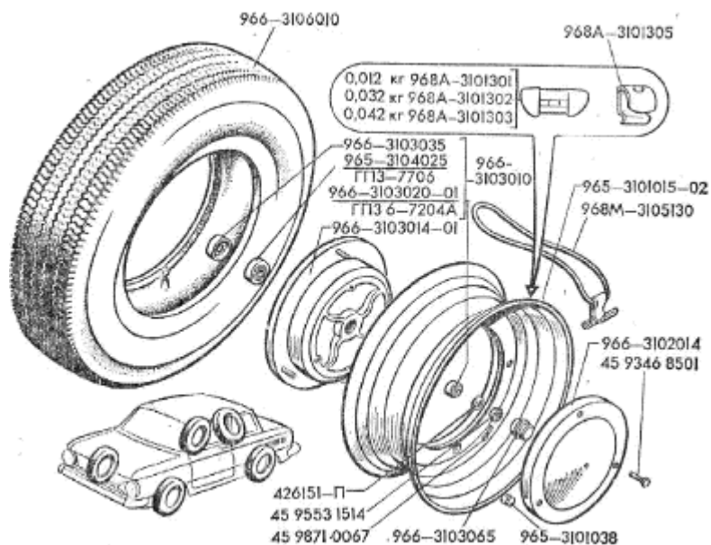
Рис.46. Колесо, колпак колеса, шина, ступица переднего колеса и держатель запасного колеса
