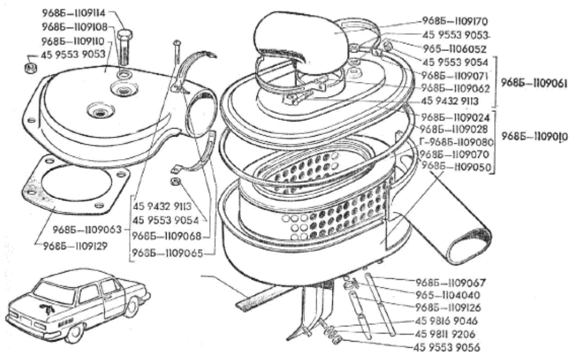
Рис.26. Фильтр воздушный сухого типа 2 von 2
