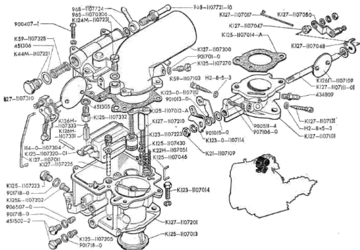
Рис.21. Детали карбюратора К-127 3 von 3
