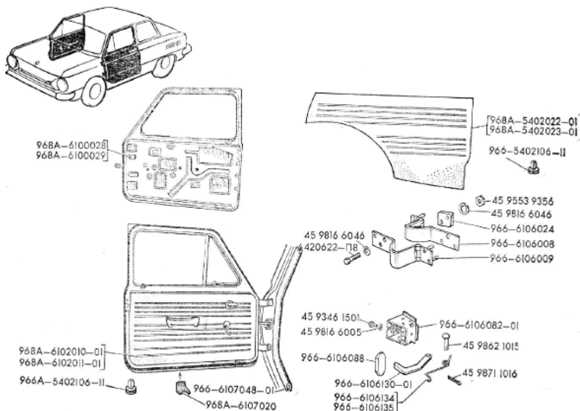
Рис.70. Дверь и обшивка боковины
