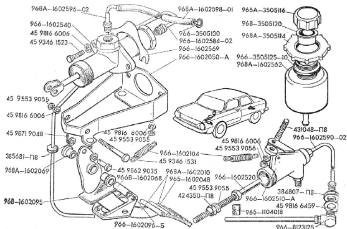
Рис.30. Привод управления сцеплением 2 von 2
