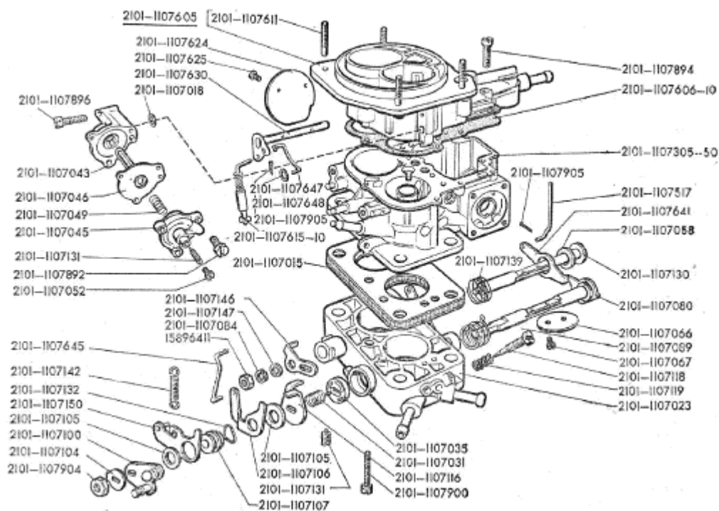
Рис.22. Детали карбюратора ДААЗ 2101-20 3 von 3
