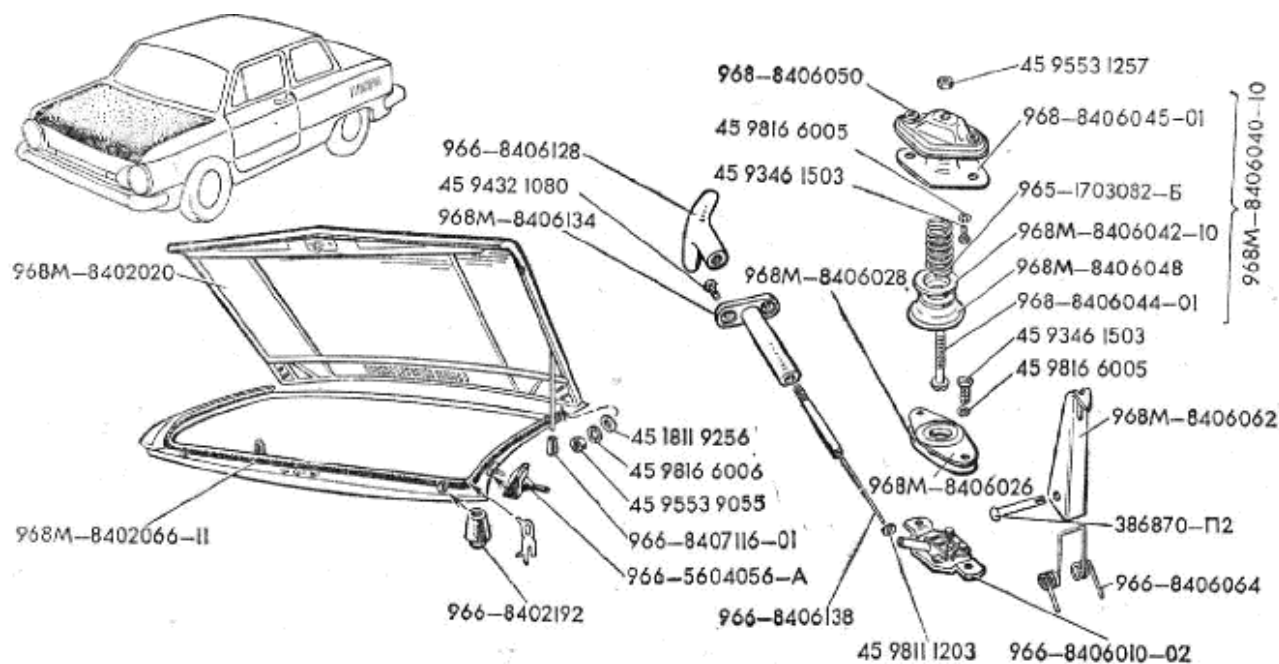
Рис.80. Капот передка
