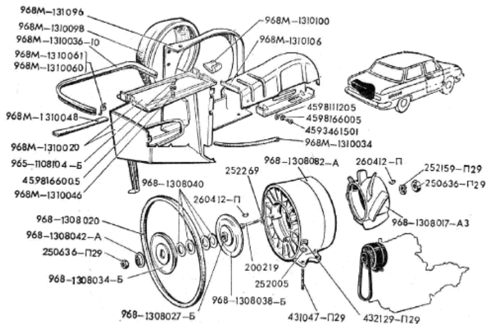
Рис.28. Детали системы охлаждения 2 von 2
