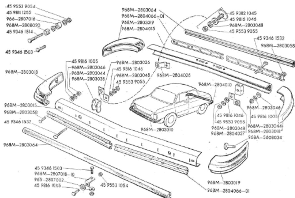
Рис.38. Буфера и крепление номерных знаков 1 von 2
