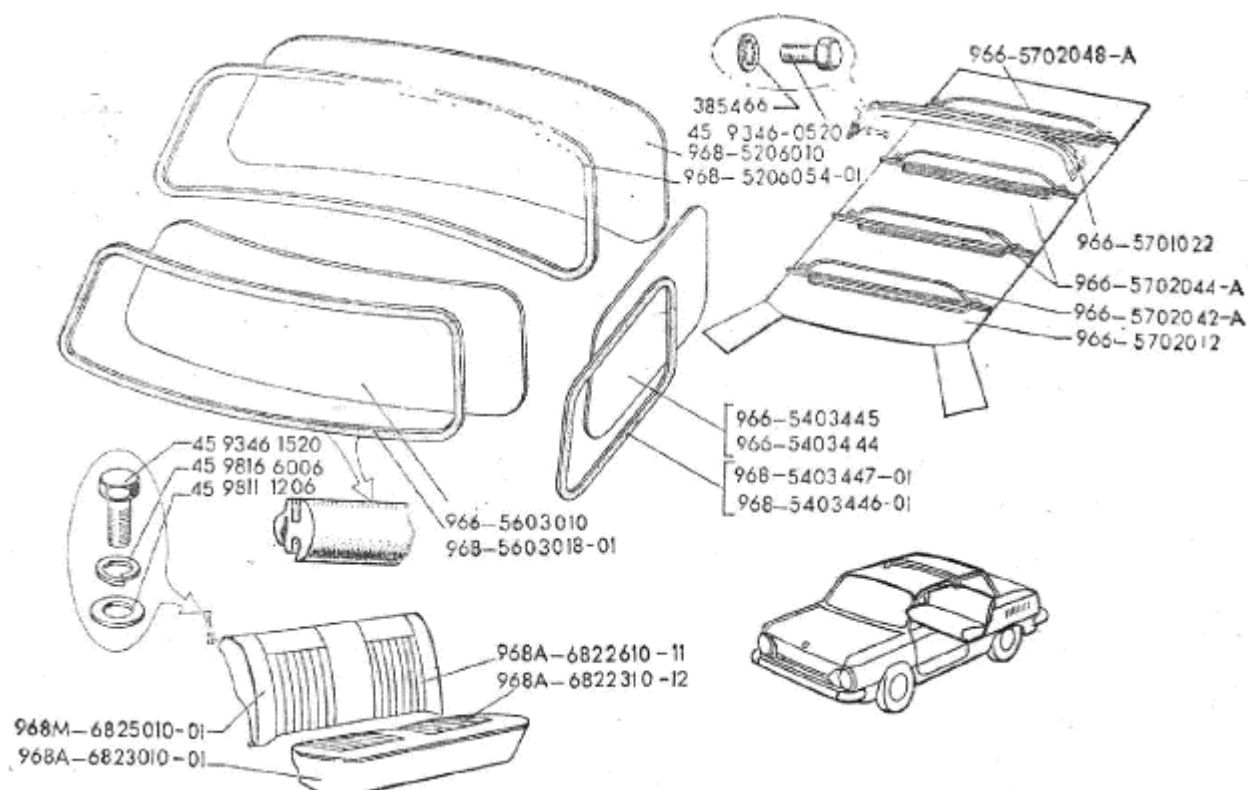
Рис.67. Стекла кузова, обивка крышки и заднее сиденье
