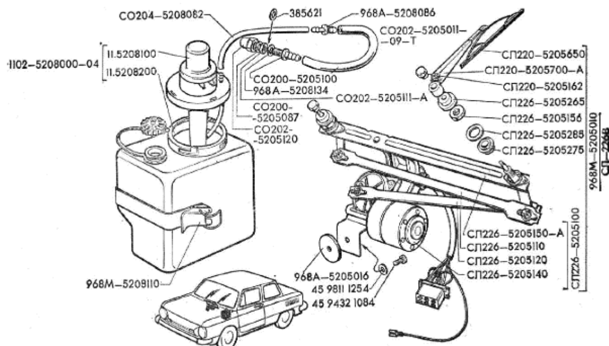
Рис.66. Стеклоочиститель и стекло омыватель
