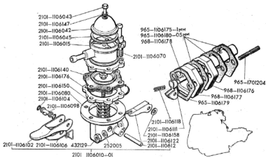
Рис.19. Топливный насос
