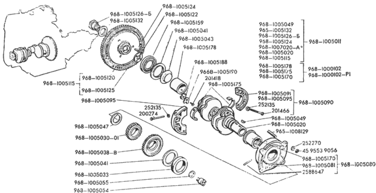
Рис. 10 Коленчатый вал и маховик
