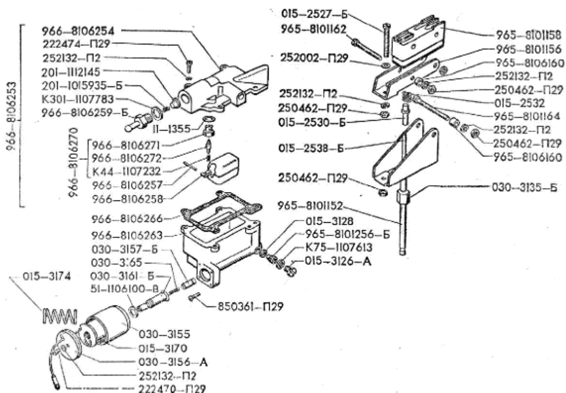
Рис.77. Детали отопительной устанавки 2 von 2
