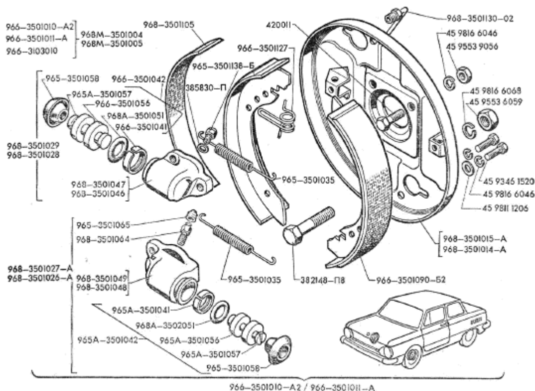
Рис.50. Передний тормоз 1 von 2
