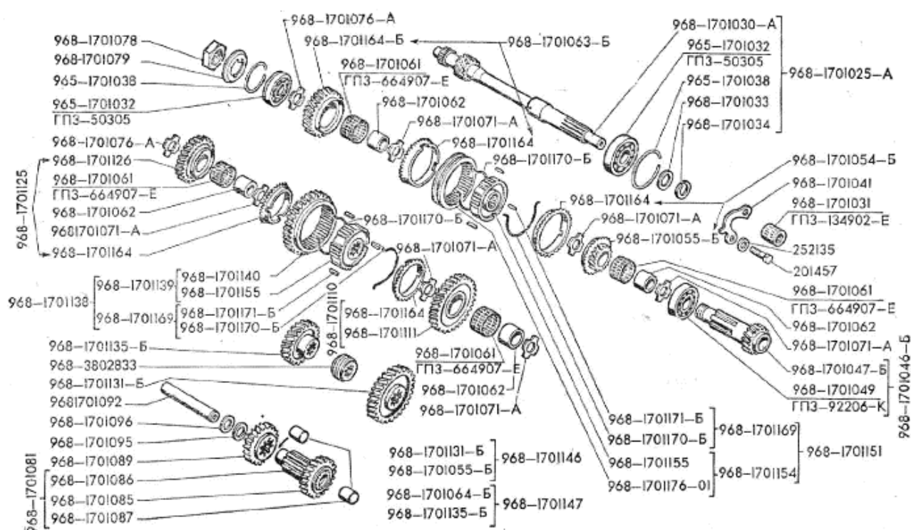
Рис.33. Детали коробки передач 3 von 4
