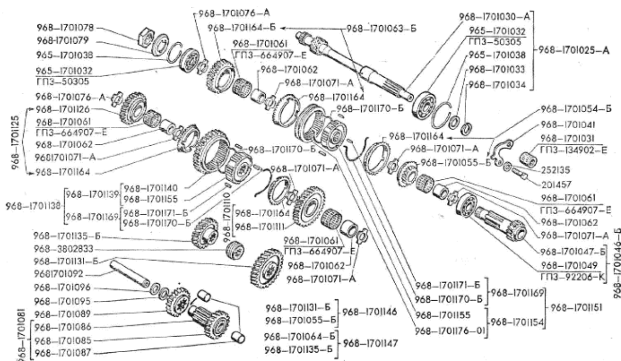
Рис.33. Детали коробки передач 1 von 4
