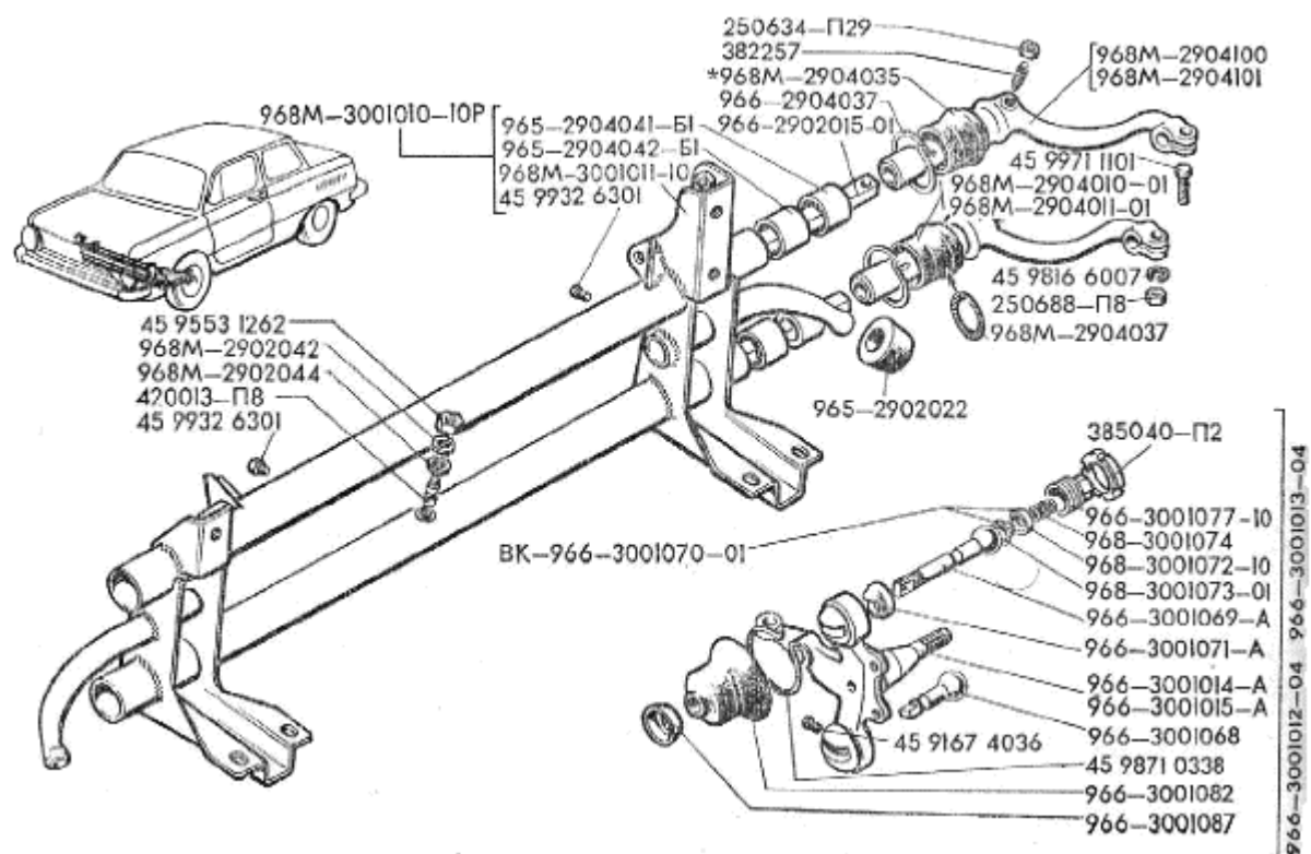
Рис.41. Детали передней подвески 3 von 3
