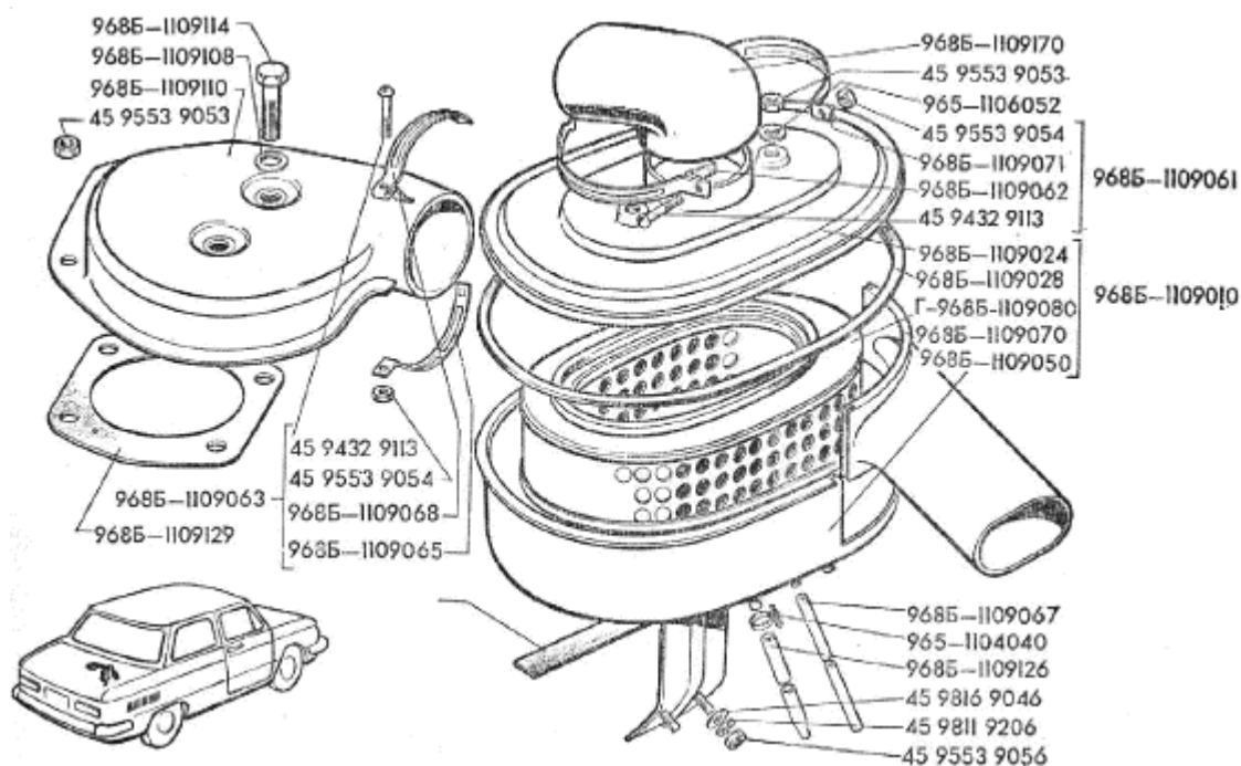
Рис.26. Фильтр воздушный сухого типа 1 von 2
