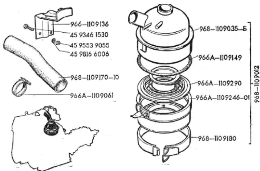
Рис.25. Фильтр воздушный инерционно-масляный
