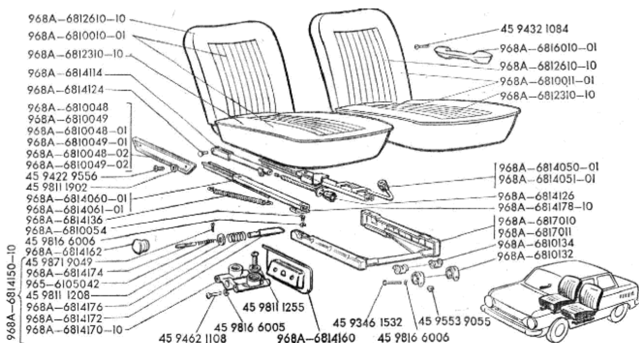
Рис.75. Переднее сиденье и подлокотник 2 von 2
