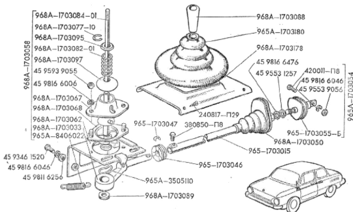
Рис.35. Механизм управления коробкой передач 1 von 2
