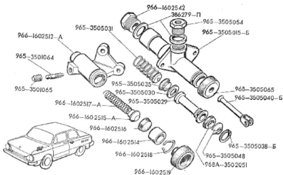
Рис.31. Детали привода управления сцеплением
