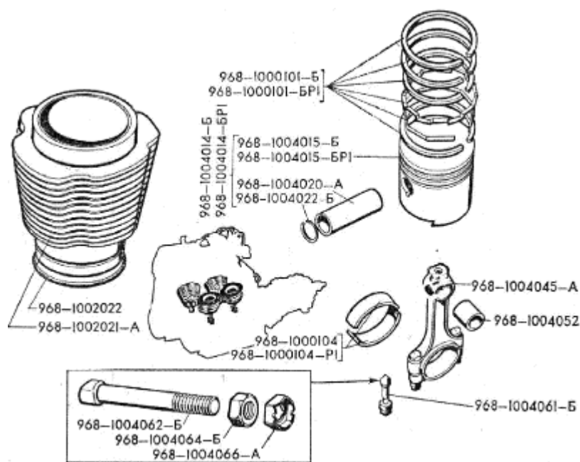
Рис. 9. Цилиндр, поршень и шатун
