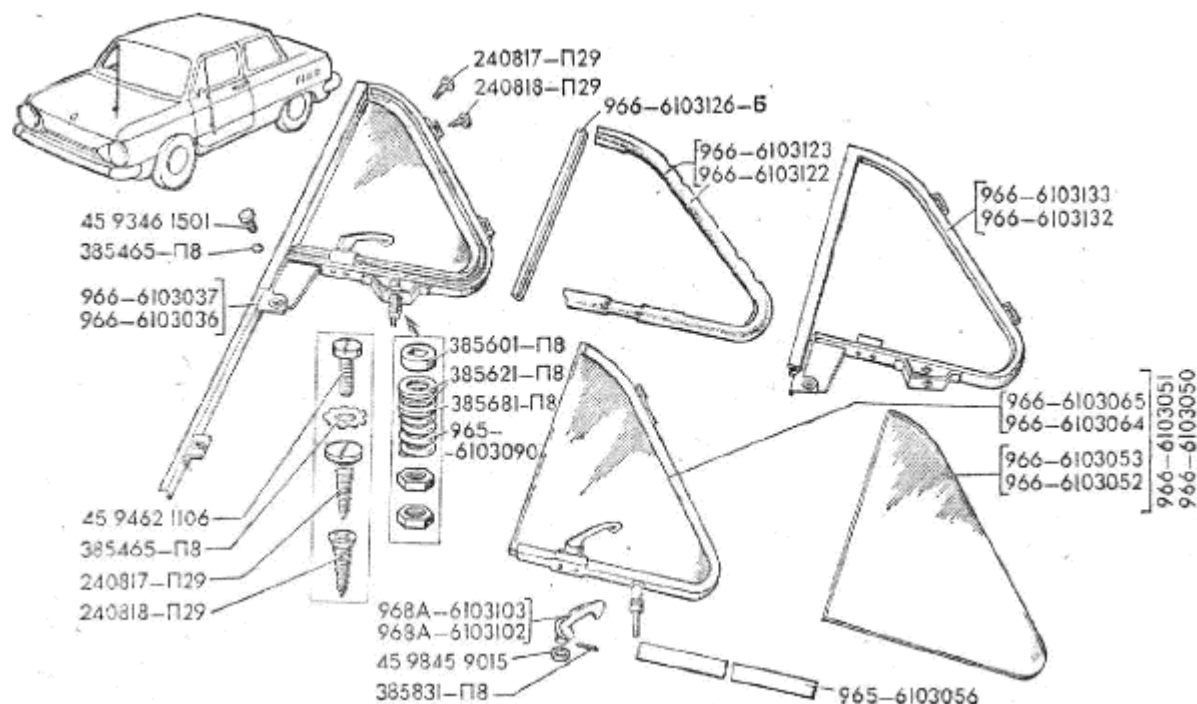
Рис.72. Поворотное стекло двери
