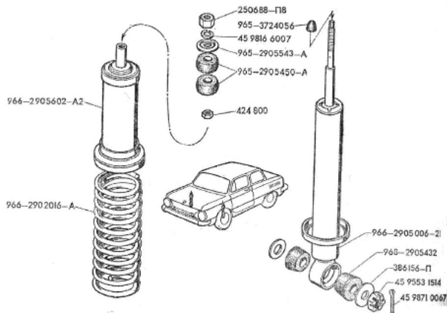
Рис.42. Амортизатор передней подвески с пружиной
