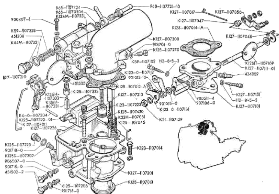
Рис.21. Детали карбюратора К-127 1 von 3
