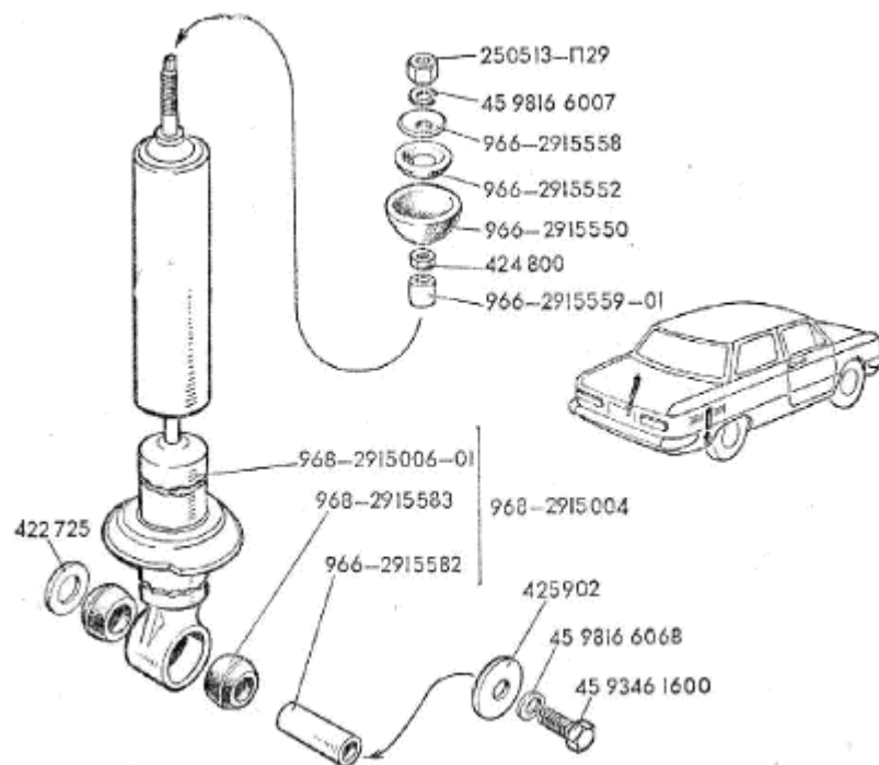
Рис.44. Амортизатор задней подвески
