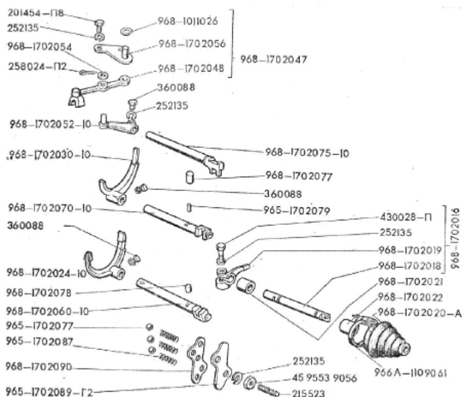
Рис.34. Детали коробки передач 2 von 2
