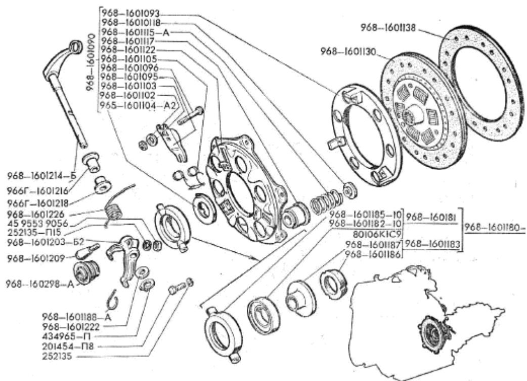
Рис.29. Механизм сцепления 2 von 2
