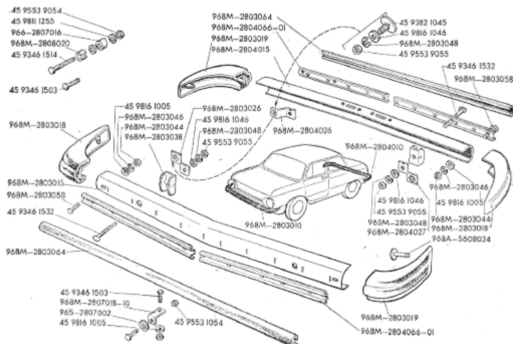
Рис.38. Буфера и крепление номерных знаков 2 von 2
