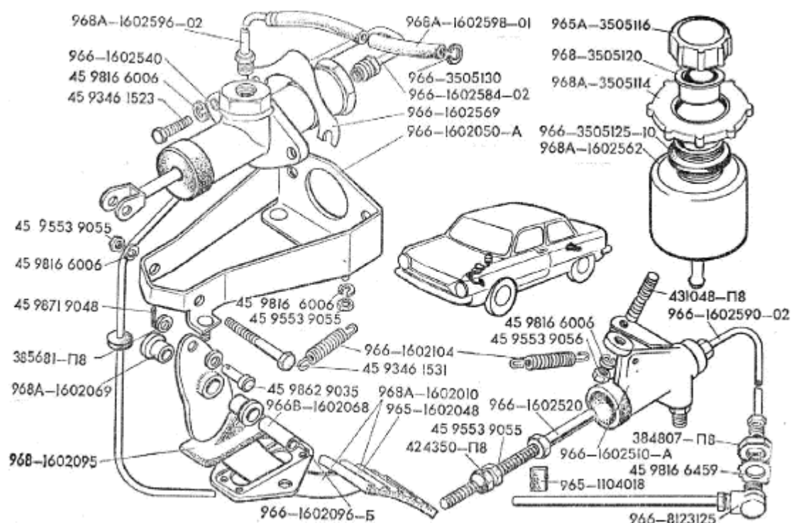
Рис.30. Привод управления сцеплением 1 von 2
