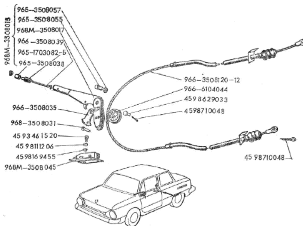
Рис.55. Управление стояночным тормозом
