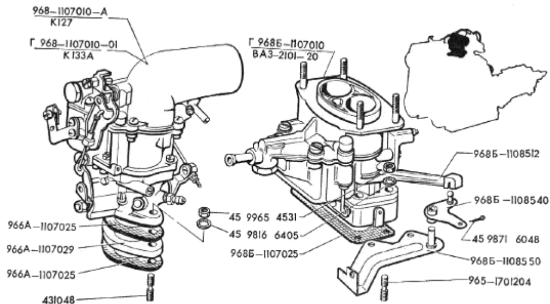
Рис.20. Карбюраторы
