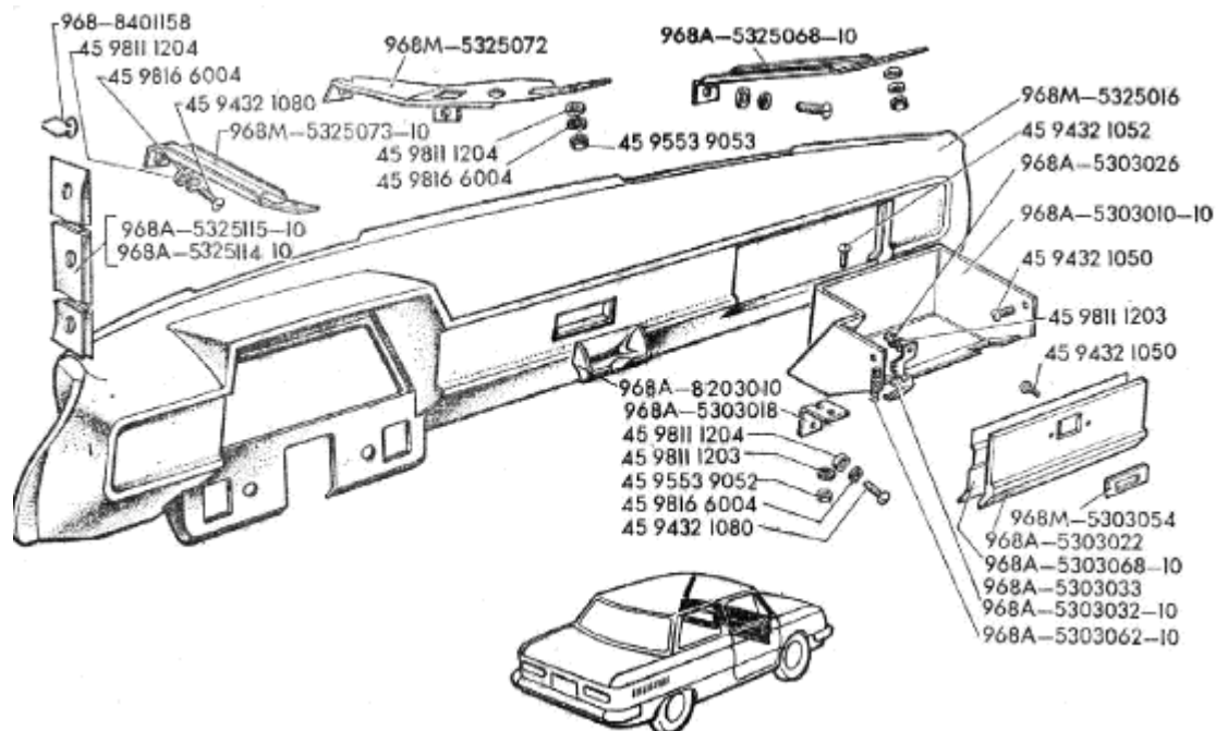
Рис.68. Панель приборов
