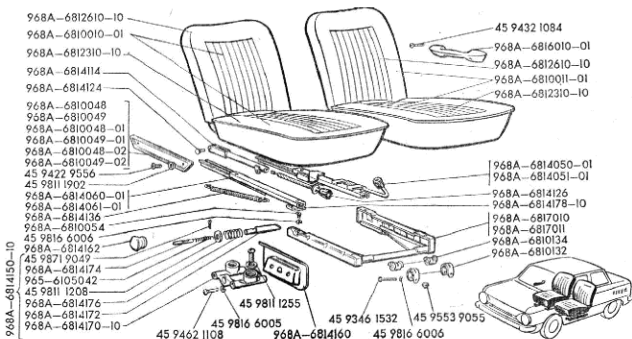
Рис.75. Переднее сиденье и подлокотник 1 von 2
