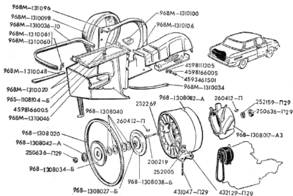
Рис.28. Детали системы охлаждения 1 von 2
