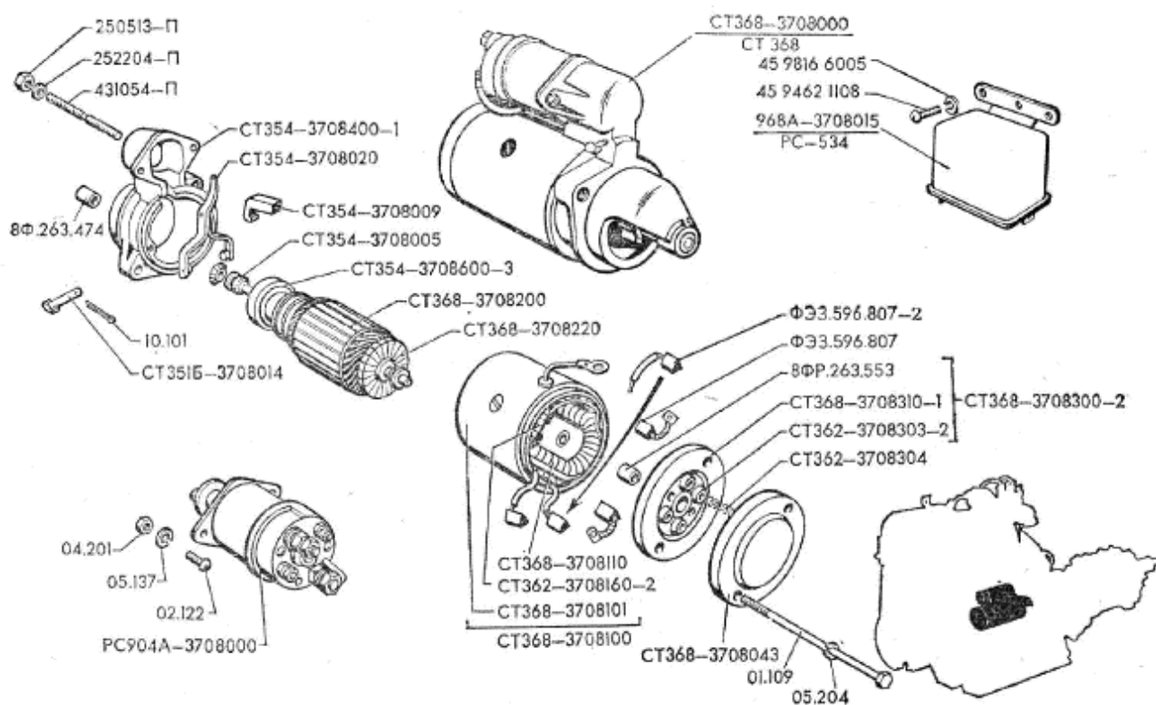
Рис.58. Стартер и включатель стартера 2 von 2
