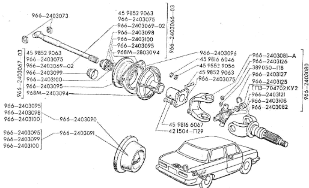
Рис.37. Полуоси
