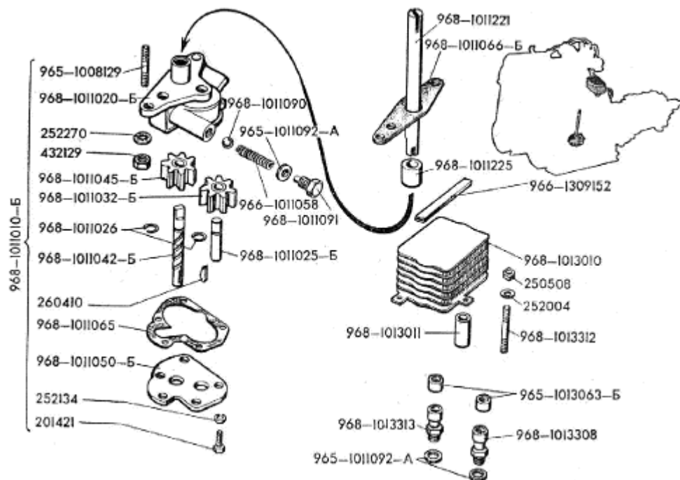
Рис. 15. Масляный насос и масляный радиатор
