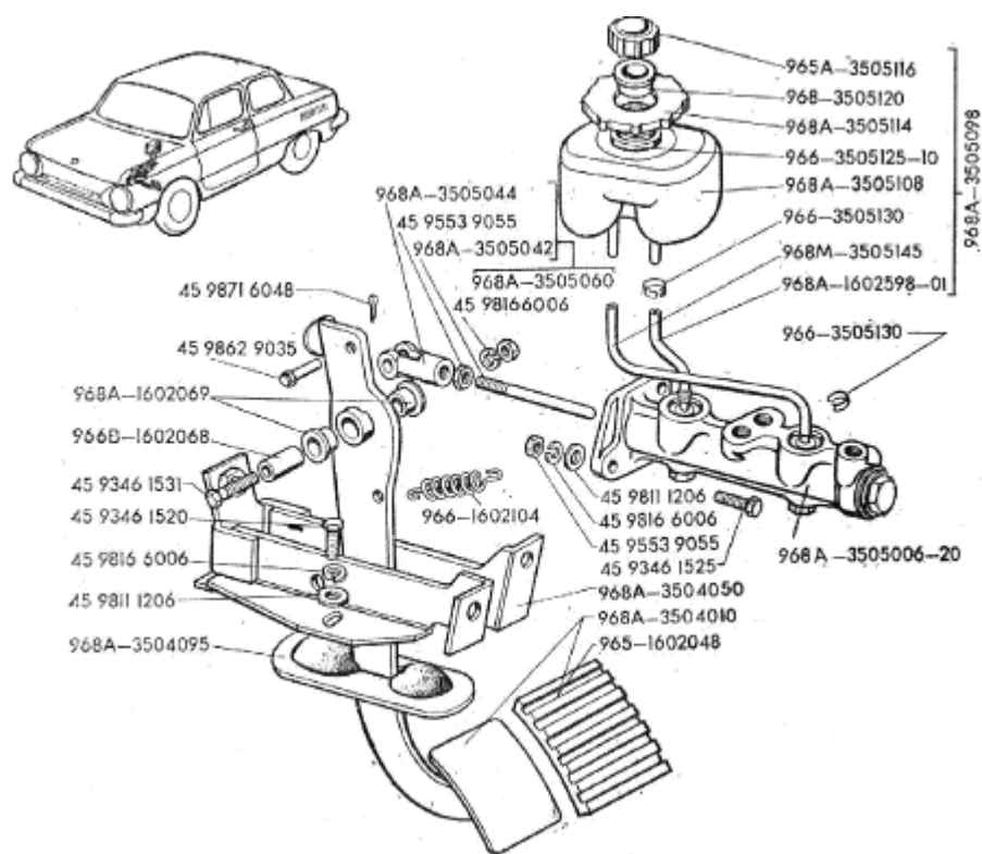
Рис.52. Привод гидравлического тормоза 1 von 2
