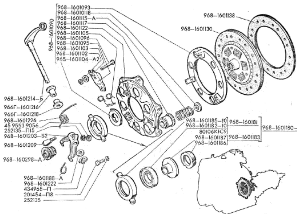
Рис.29. Механизм сцепления 1 von 2
