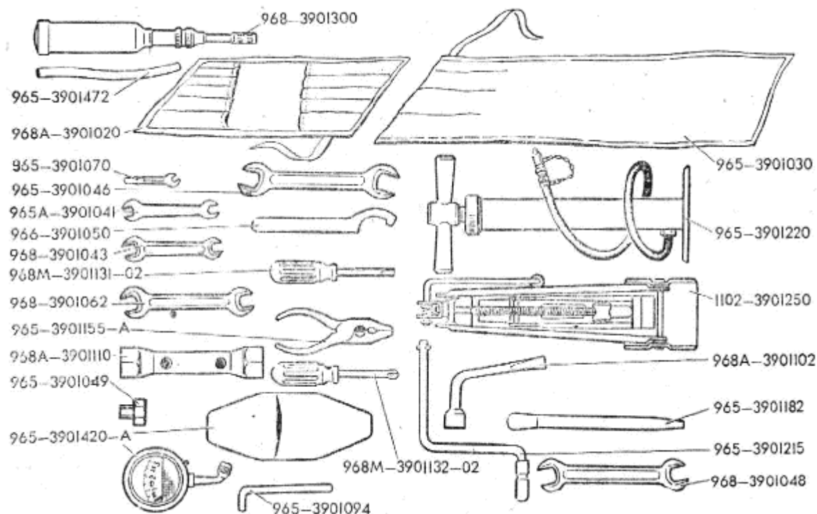
Рис.63. Инструмент
